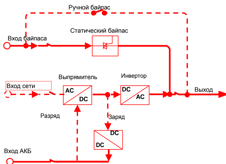
Рис 2-11 Режим работы через байпас ((жирная линия показывает поток энергии))
