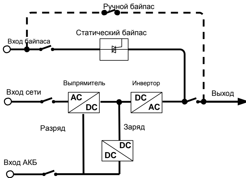
Рис. 2-8 Функциональная диаграмма
