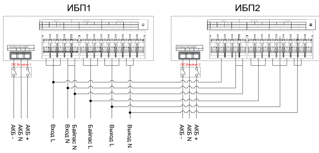
Рис. 3-28 10/10S/15/15S/20/20S диаграмма подключения для 11 режима параллельной системы
