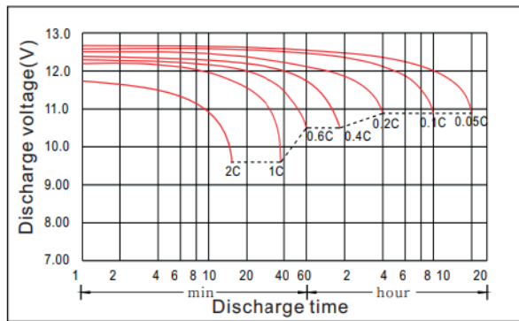
Разрядная характеристика
